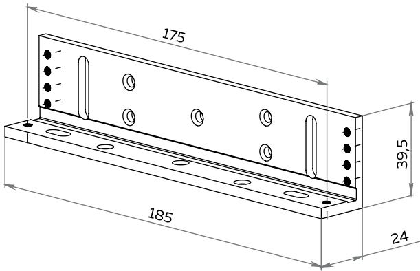
поз. 3 — Монтажный уголок
