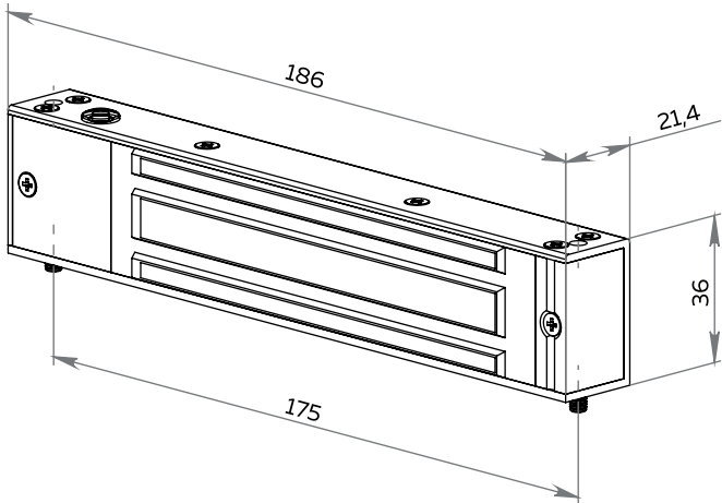
поз. 1 — Электромагнит
