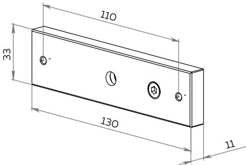
поз. 4 — Ответная планка
