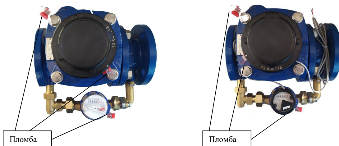
Рисунок А5. Внешний вид и опломбировка счётчиков КВСХ-05, КВСХд-05.
