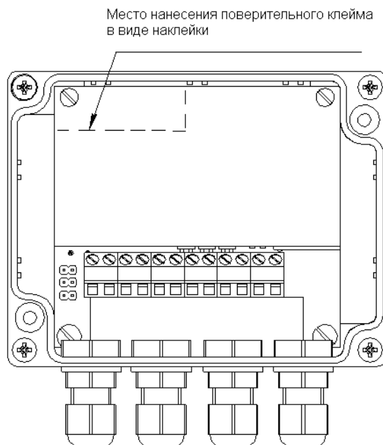
Рис. 1в. Пломбирование
