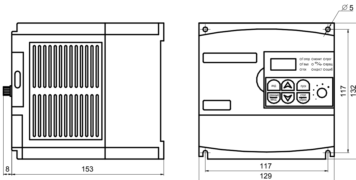
Преобразователь ЕЗ-8100В-002Н
