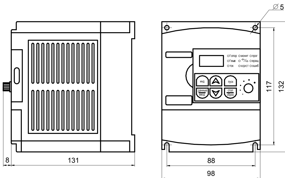
Преобразователь ЕЗ-8100В-002Н
