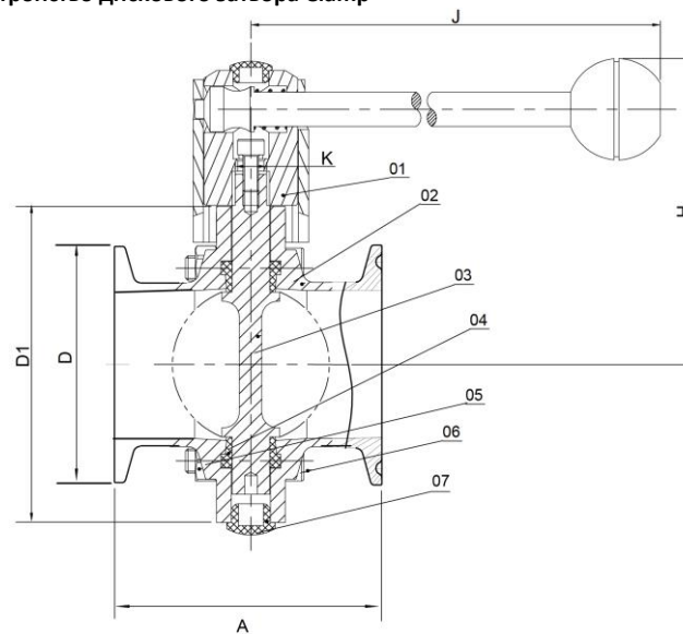
Рис. 1. Устройство дискового затвора Clamp
