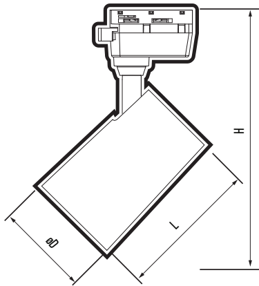
Рис 1. Прожектор PTR 07
