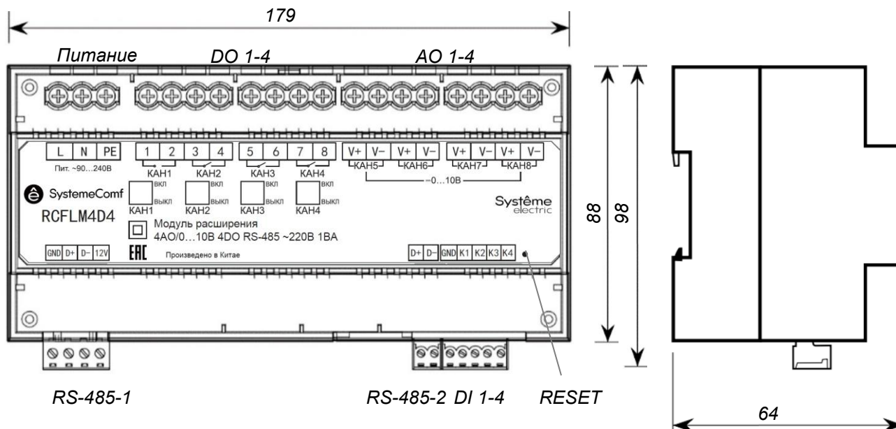
Модуль управления освещением RCFLM4, размеры в мм
