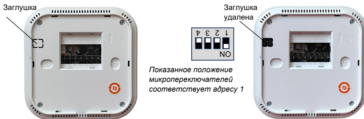
Расположение заглушки и микрпереключателей установки адреса
