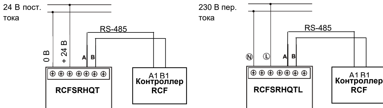
Схема подключения датчиков RCFSRHQT, RCFSRHQTL
