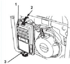
Рис.9. Снятие воздушного фильтра
