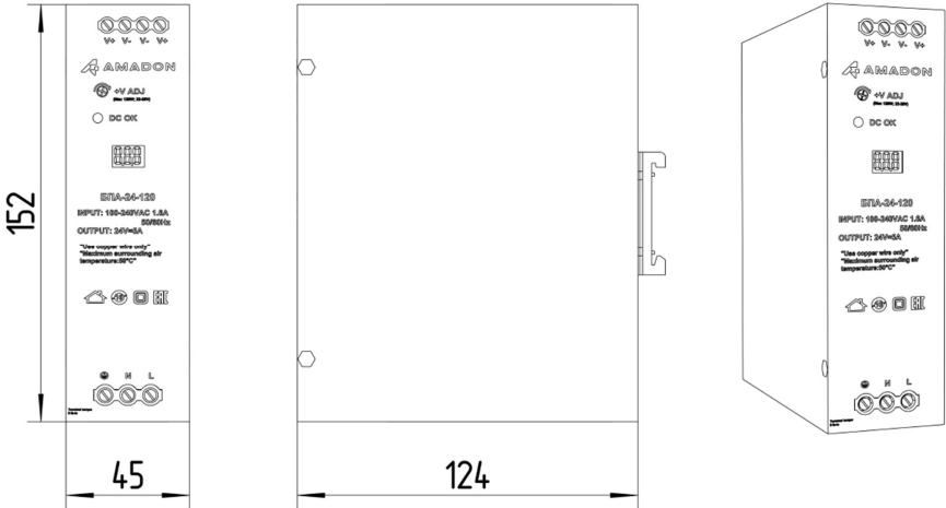
Рис. 1. Внешний вид и габаритные размеры
