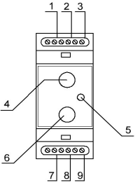
Рис. 2. Вид спереди. 1. Клеммы аварийного термостата (70 град). 2. Клеммы подключения аппаратуры. 1. 3. Клемма подключения аппаратуры. 2. 4. Регулятор значения температуры канала аппаратуры. 5. Индикатор питания. 6. Регулятор значения температуры канала обогрева. 7. Клеммы питания 230В 50 Гц. 8. Клеммы Подключения обогревателя. 1. 9. Клеммы подключения обогревателя. 2.
