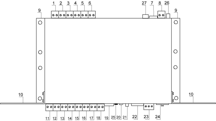
Рис.1 Вид спереди. 1. Клеммы выхода PB1. 2. Клеммы выхода PB2. 3. Клеммы выхода PB3. 4. Клеммы выхода PB4. 5. Клеммы выхода PB5. 6. Клеммы выхода PB6. 7. Гнездо питания 5,5х2,1. 8. Клемма питания винтовая. 9. Кронштейн консольного крепления. 10. Кронштейн крепления к стойке 19 дюймов (отделяемый). 11. Клеммы дискретного входа Ц1. 12. Клеммы дискретного входа Ц8. 13. Клеммы дискретного входа Ц7. 14. Клеммы дискретного входа Ц6. 15. Клеммы дискретного входа Ц5. 16. Клеммы дискретного входа Ц4. 17. Клеммы дискретного входа Ц3. 18. Клеммы дискретного входа Ц2. 19. Гнездо цифрового входа Ц1. 20. Индикатор питания. 21. Кнопка сброса. 22. Гнездо подключения /BС (Ethernet). 23. Клемма подключения RS-485. 24. Крышка гнезда для установки SIM-карты (для УМА-5ИС). 25. Переключатель безопасности. 26. Винт заземления. 27. Гнездо подключения внешней антенны (для УМА-5ИС).
