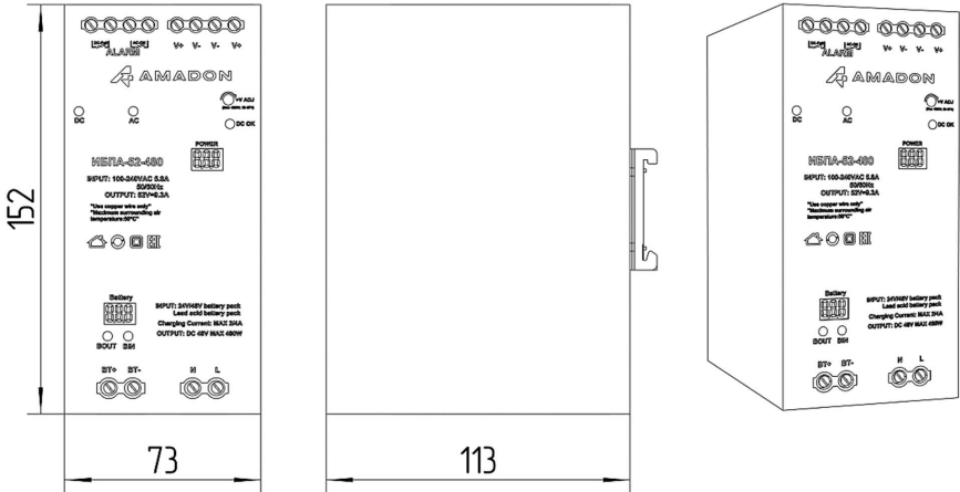
Рис. 1. Внешний вид и габаритные размеры.
