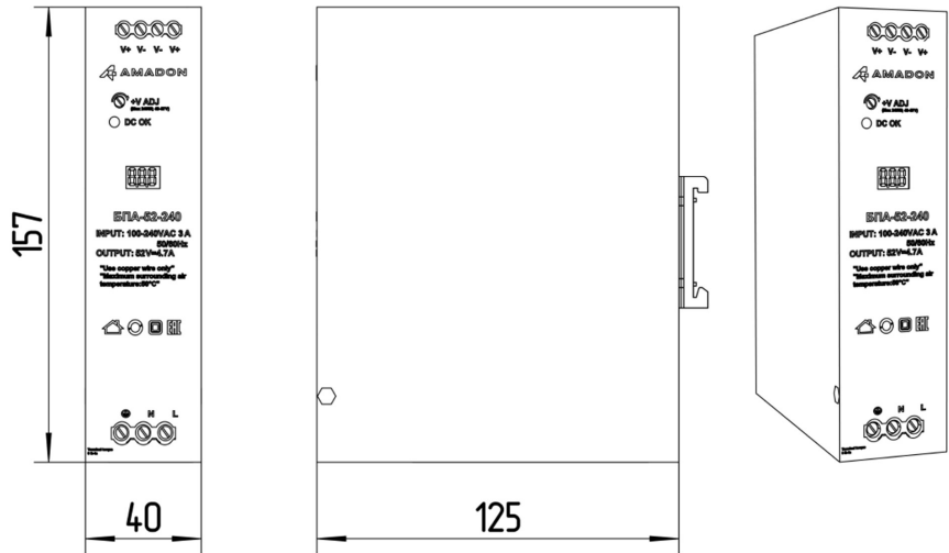
Рис. 1. Внешний вид и габаритные размеры.
