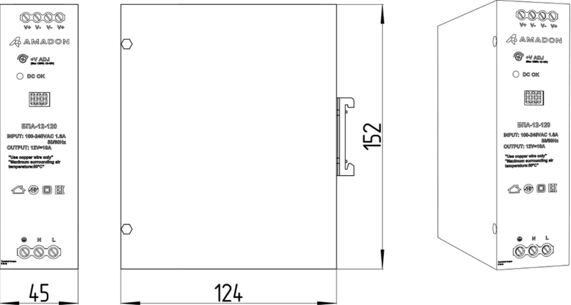
Рис. 1. Внешний вид и габаритные размеры.
