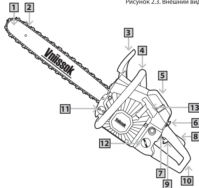
Рисунок 2.3. Внешний вид
