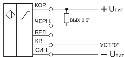
Схема подключения
