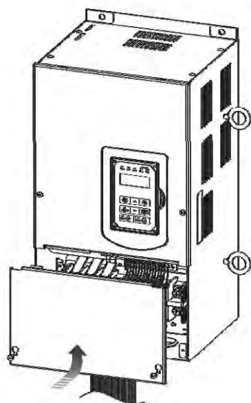
Шаг3: подключить провода и поставить крышку на место
