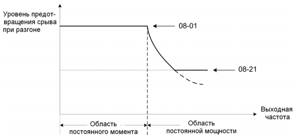
Уровень и ограничение предотвращения срыва при разгоне.
