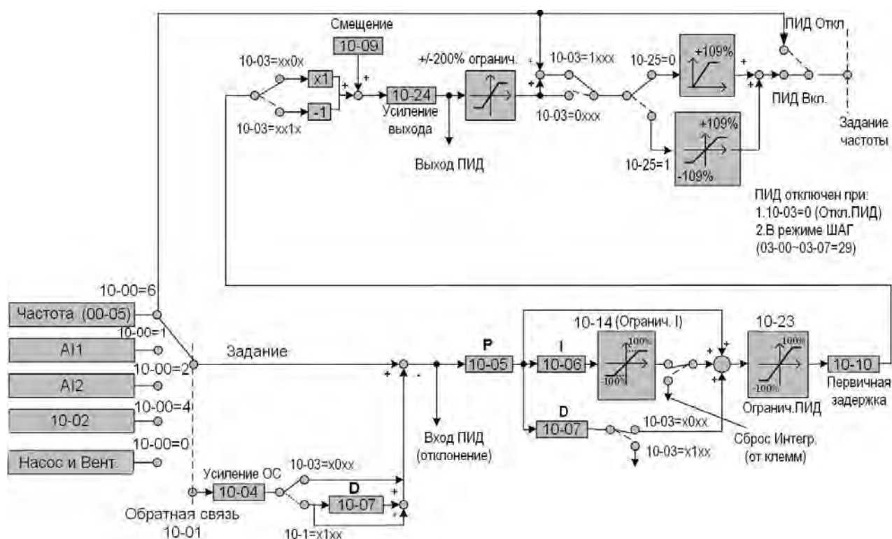
Блок-схема ПИД-регулятора
