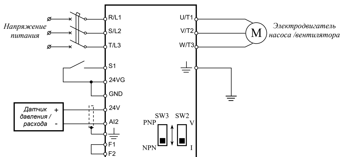
Схема подключения E5-P7500 для работы в режиме ПИД-регулирования.
