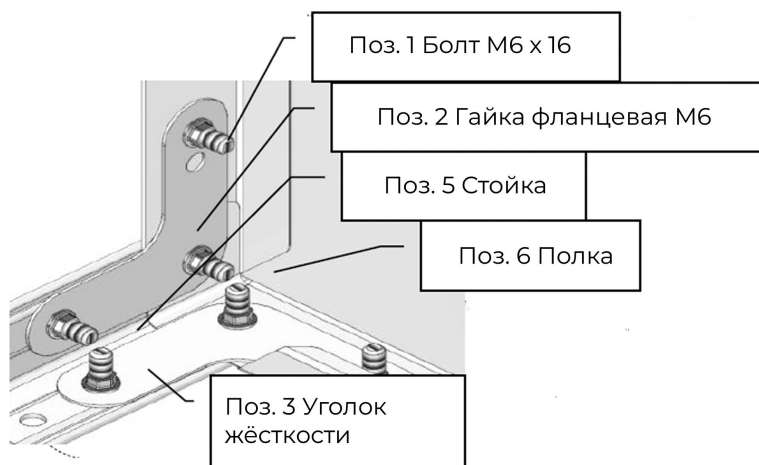
Крепление полок с уголком жёсткости
