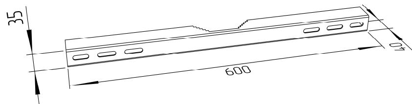
Рис. 2. Кронштейн на шкаф. 2 единицы. Маркировка КМАЗ-01.
