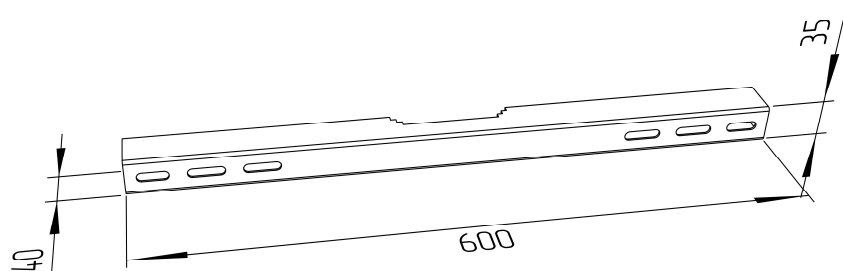
Рис. 3. Кронштейн на стол. 2 единицы. Маркировка КМАЗ-02.
