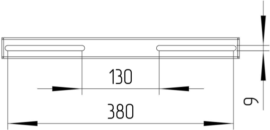
Рис. 1. Расстояния, в пределах которых можно закрепить оборудование.
