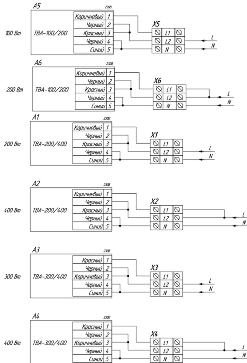
Рис. 2. Варианты подключения.
