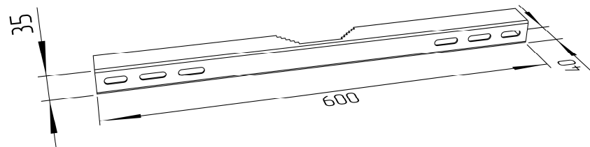
Рис. 2. Кронштейн на шкаф. 2 единицы. Маркировка КМАЗН-01.
