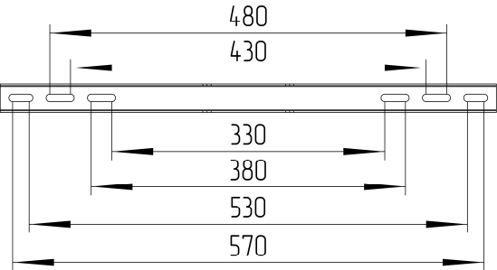
Рис. 1. Расстояния, в пределах которых можно закрепить оборудование.
