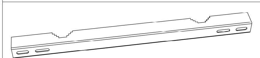
Рис. 2. Кронштейн на шкаф. 2 единицы. Маркировка КМАЗ-1Н-01.
