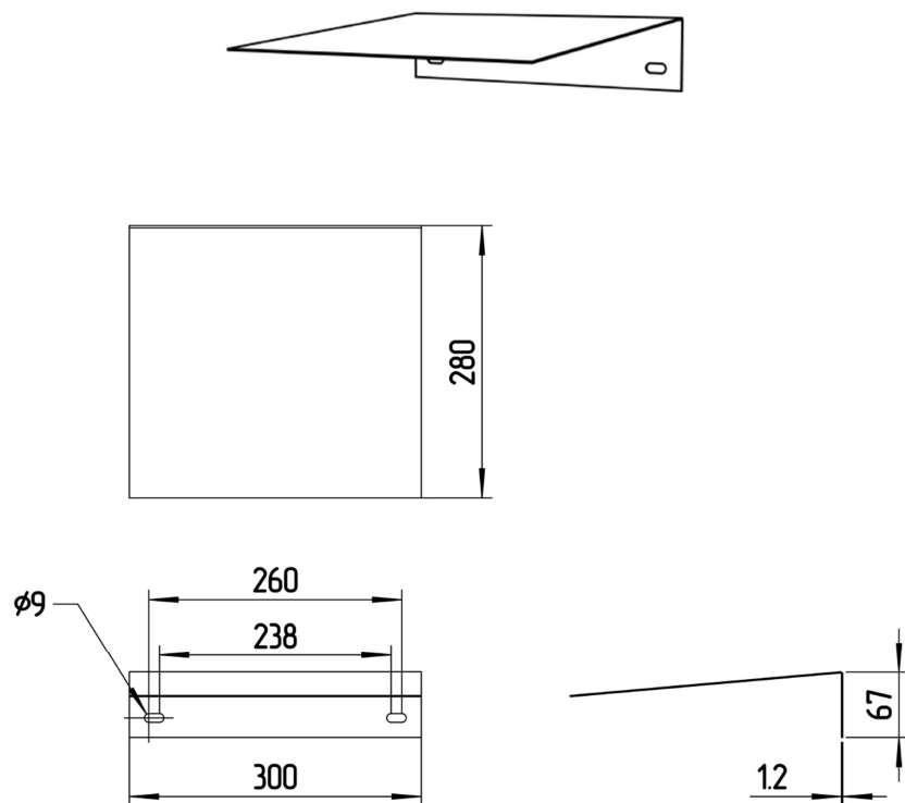
Рис. 1. Внешний вид и габаритные размеры.
