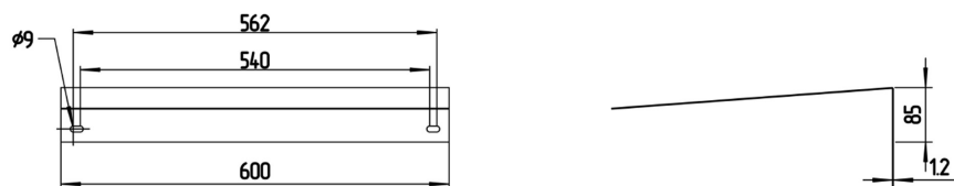
Рис. 1. Внешний вид и габаритные размеры.
