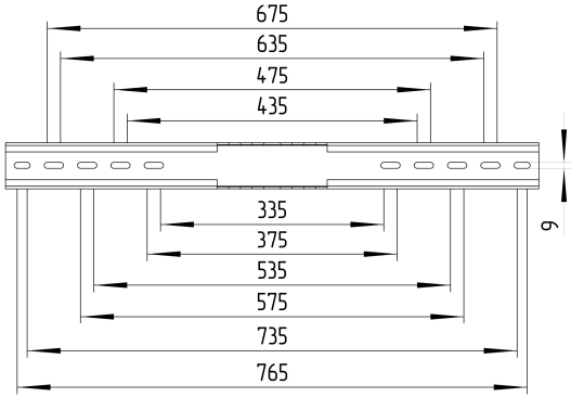
Рис. 1. Расстояния, в пределах которых можно закрепить оборудование.
