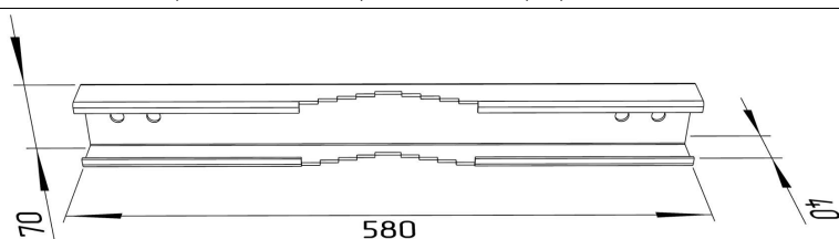
Рис. 3. Кронштейн на опору. 2 единицы. Маркировка КМА4Н-02.
