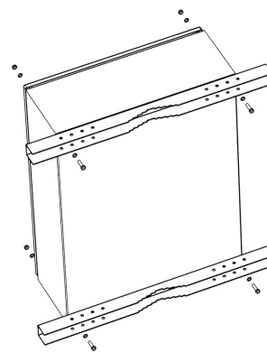
Рис. 13. Закрепить кронштейны КМА4Н-01 к шкафу.
