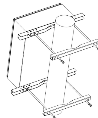
Рис. 16. Зафиксировать на кронштейн КМА4Н-02.
