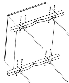
Рис. 15. Закрепить шпильки на кронштейн.
