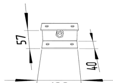
Рис. 5. Переходник на шпильку. 4 единицы. Маркировка КМА4Н-03.
