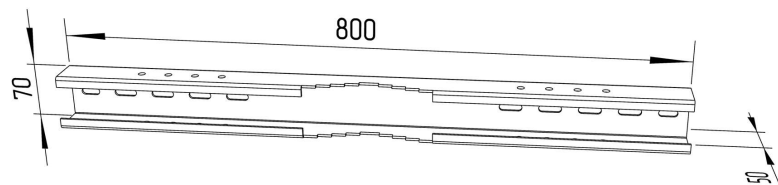
Рис. 2. Кронштейн на шкаф. 2 единицы. Маркировка КМА4Н-01.
