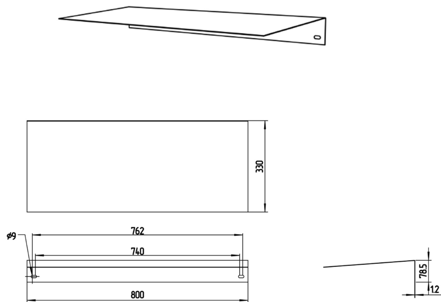
Рис. 1. Внешний вид и габаритные размеры.
