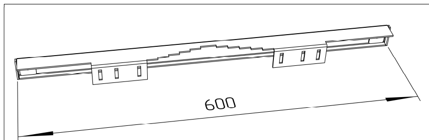
Рис. 2. Крепление на шкаф. 2 единицы. Маркировка КМА2Н.
