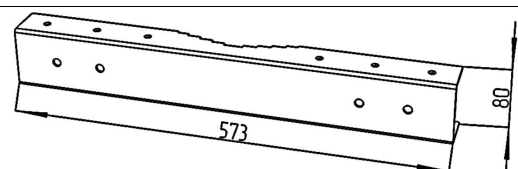
Рис. 2. Кронштейн на шкаф. 1 единица. Маркировка КМА-4А-Х-01.
