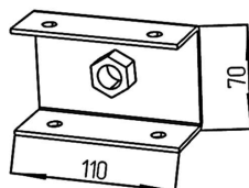
Рис. 5. Переходник на шпильку. 2 единицы. Маркировка КМА-4А-Х-03.
