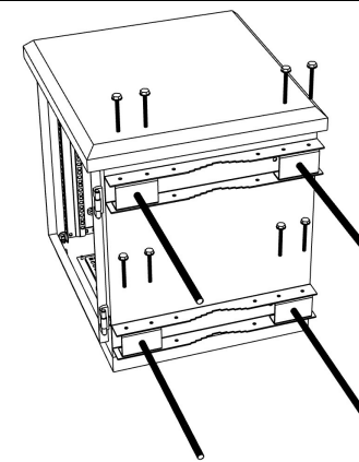
Рис. 14. Закрепить шпильки на кронштейн.
