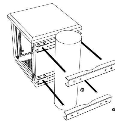
Рис. 15. Зафиксировать на кронштейн КМА-4А-Х-02.
