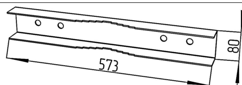
Рис. 3. Кронштейн на опору. 1 единица. Маркировка КМА-4А-Х-02.
