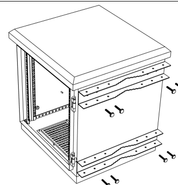
Рис. 12. Закрепить кронштейны КМА-4А-Х-01 к шкафу.
