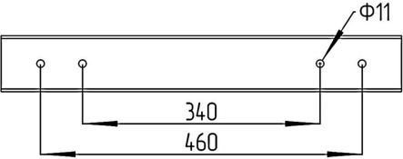
Рис. 1. Расстояния, в пределах которых можно закрепить оборудование.
