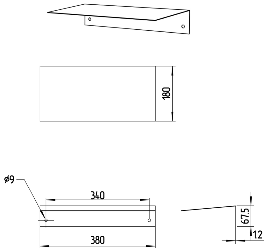
Рис. 1. Внешний вид и габаритные размеры.
