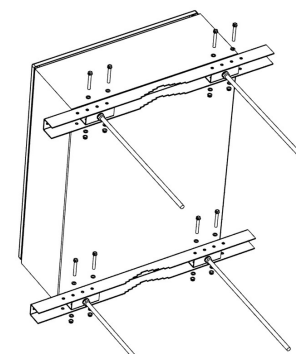
Рис. 13. Закрепить кронштейны КМА4-01 к шкафу.
