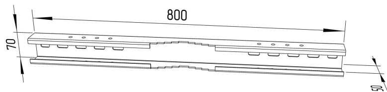
Рис. 2. Кронштейн на шкаф. 2 единицы. Маркировка КМА4-01.
