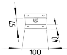
Рис. 5. Переходник на шпильку. 4 единицы. Маркировка КМА4-03.
