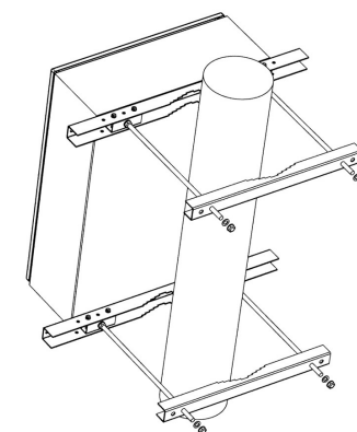
Рис. 16. Зафиксировать на кронштейн КМА4-02.
