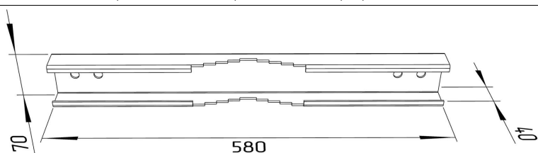
Рис. 3. Кронштейн на опору. 2 единицы. Маркировка КМА4-02.
