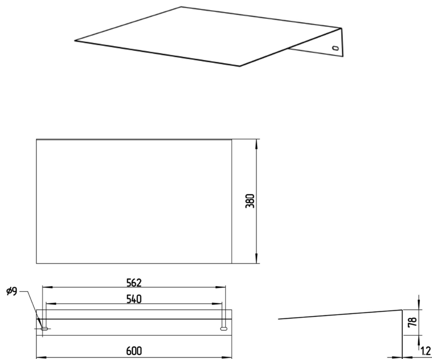
Рис. 1. Внешний вид и габаритные размеры.
