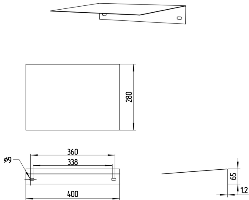
Рис. 1. Внешний вид и габаритные размеры.
