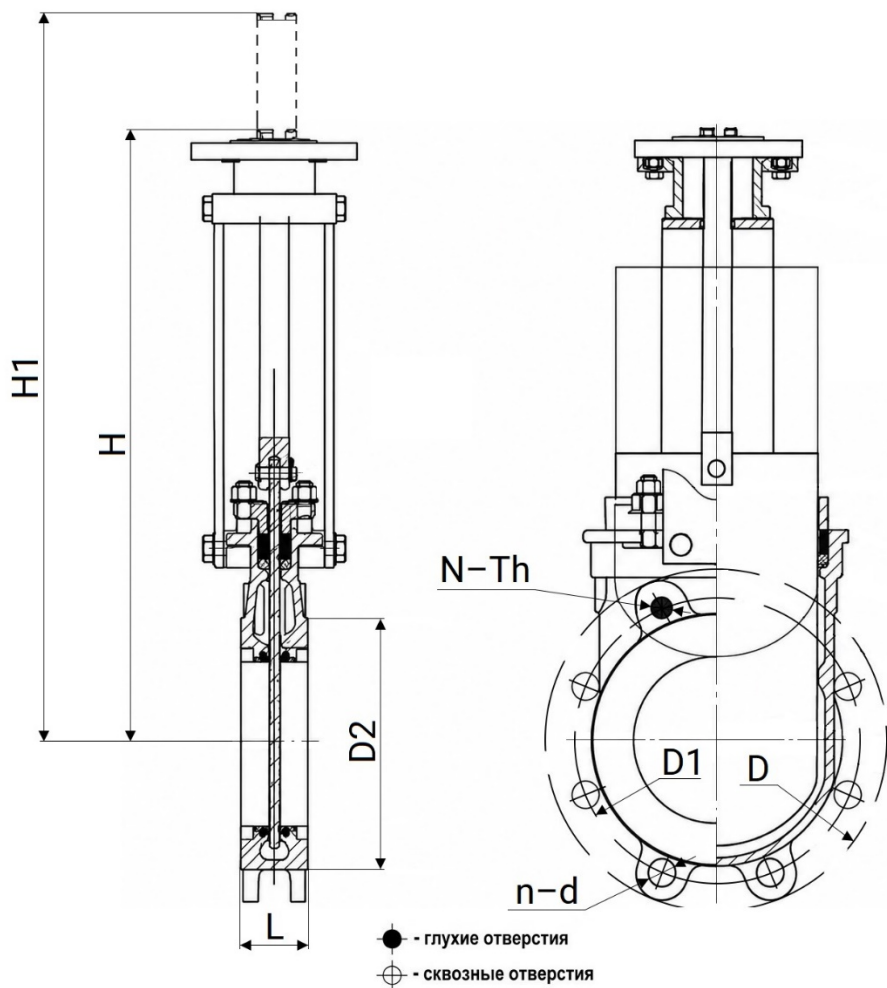
Рисунок 3 – Размеры изделия
