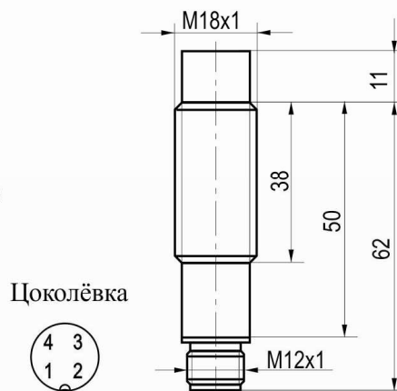
Габаритный чертеж
