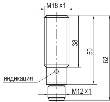
Габаритный чертеж
