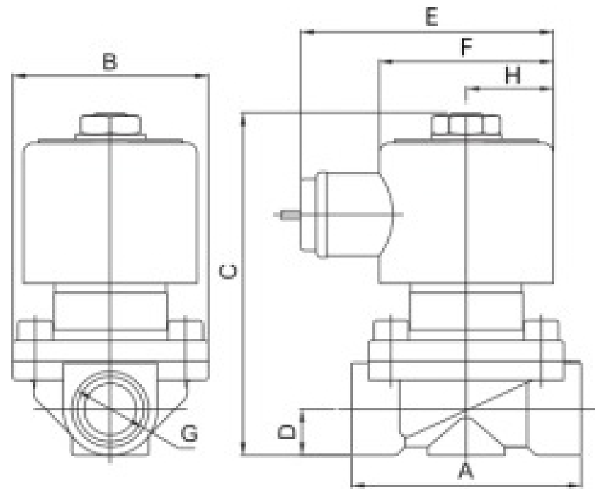
Табл.1 Размеры
