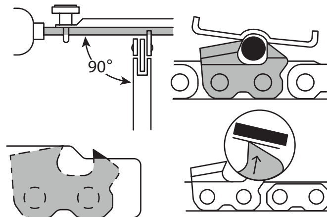
Рисунок 3.1.1. Заточка цепи
