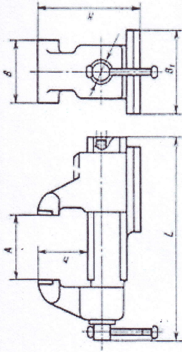
Рис. 1. Тиски слесарные неповоротные облегченные
