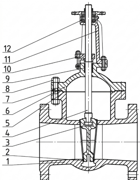
Рисунок 2 – Составные части изделия
