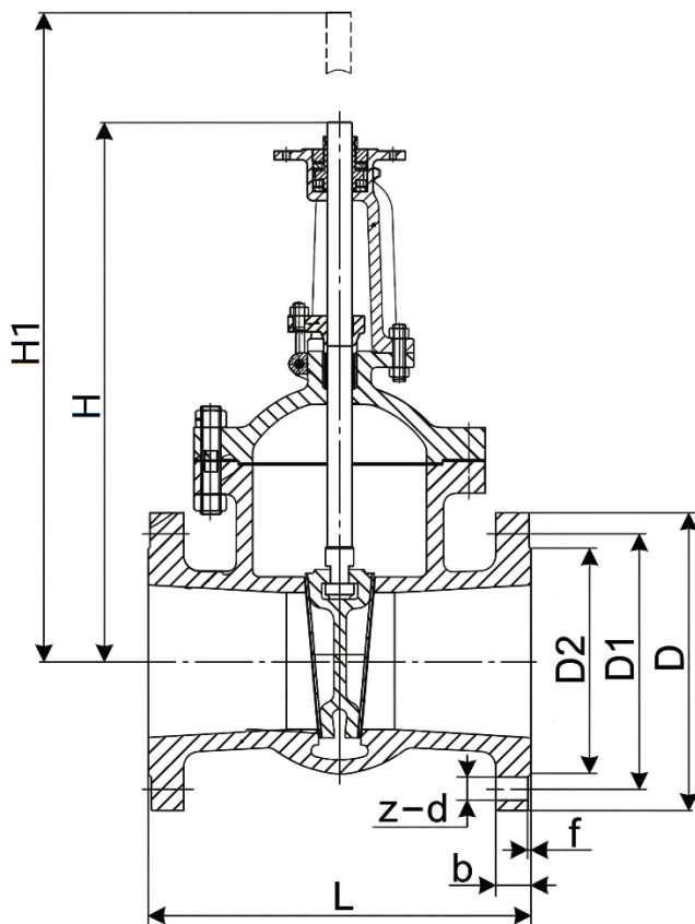
Рисунок 3 – Размеры изделия
