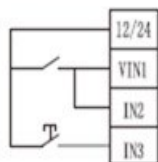
Двухпроводная схема подключения
