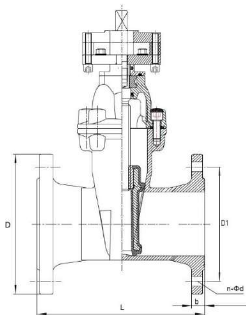
Рисунок 2 - Размеры
