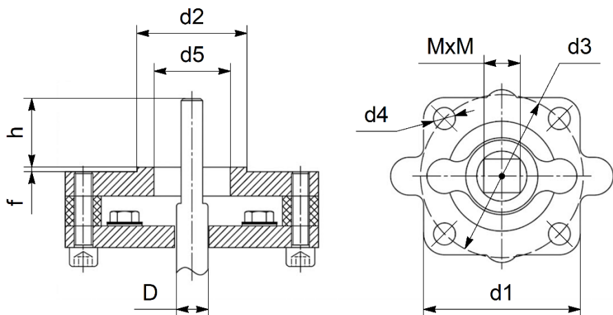
Рисунок 4 – Размеры ОСТ фланца
