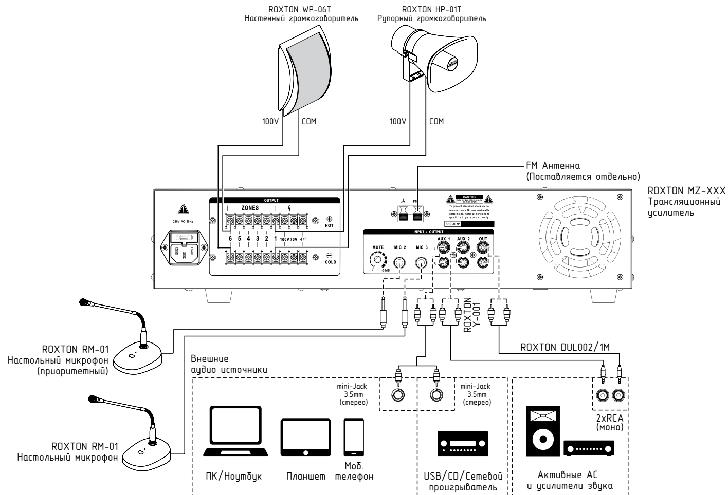
Рисунок В.1 Схема подключения ROXTON MZ-120, MZ-240, MZ-360
