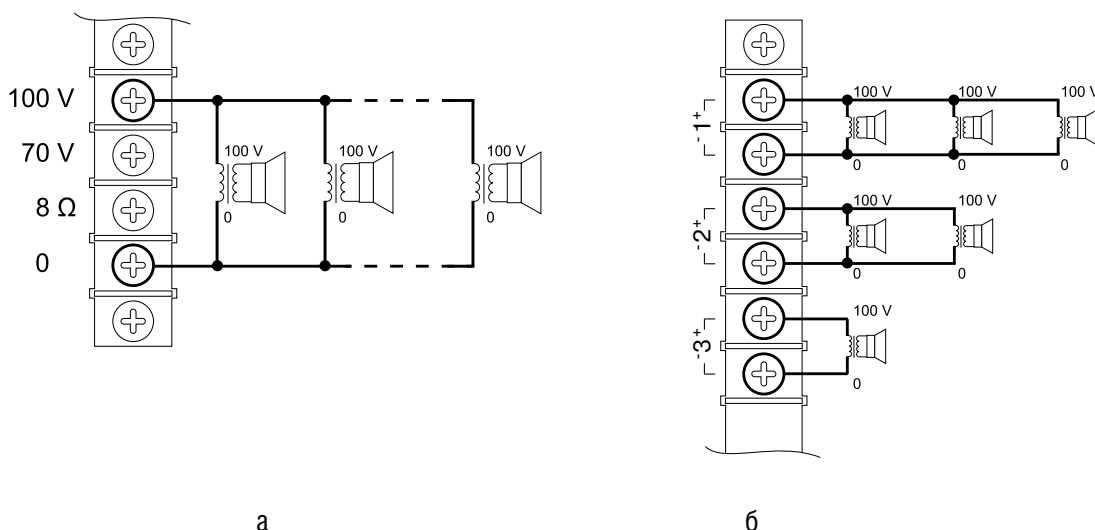
Рисунок 9.3 Схема подключения трансляционных громкоговорителей: а - напрямую; б - через селектор зон
