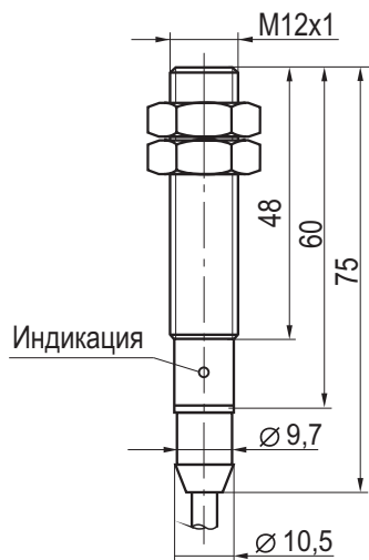
Габаритный чертеж
