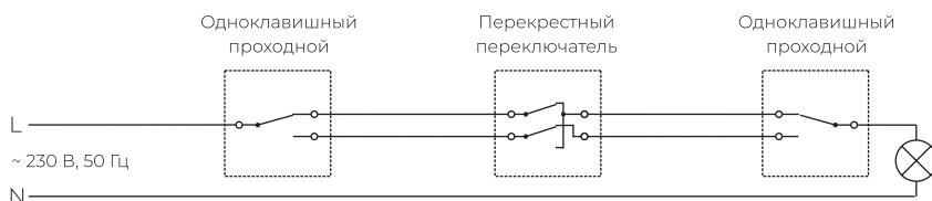
Схема управления светом из трех точек
