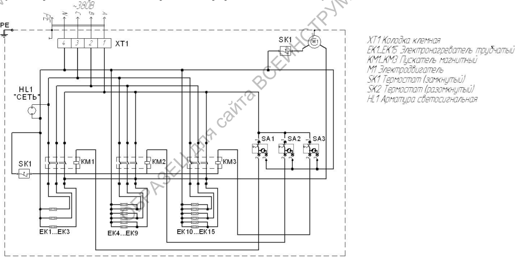
Рис. 2 Схема электрическая принципиальная
