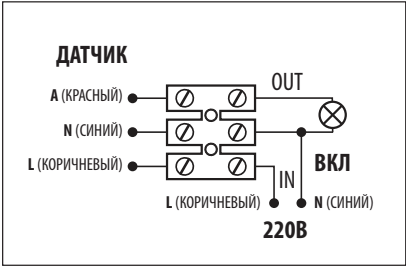
Рис 1. Схема подключения датчика
