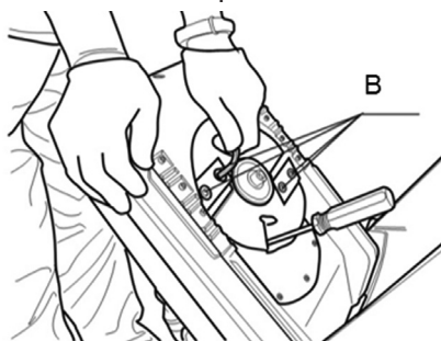
Рис. 9. Снятие ножей
